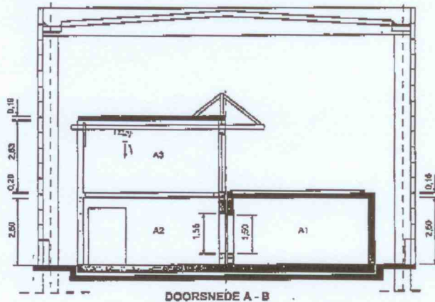
GEBOUW K: Meetcel A1 Geluidsoverdracht van contactgeluiden
